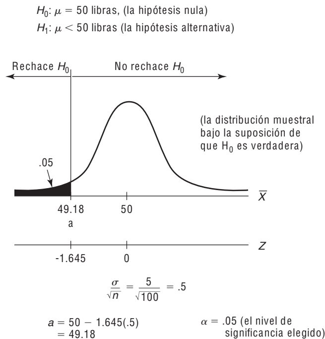
FIGURA 2-10 Prueba de hipótesis para el ejemplo 2.8
