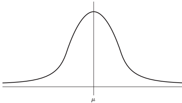
FIGURA 2-6 Una distribución normal
