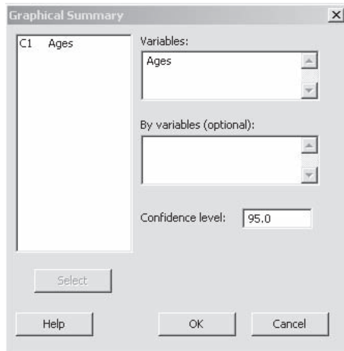
FIGURA 2-20 Pantalla de Minitab de la ventana de diálogo Graphical Summary
