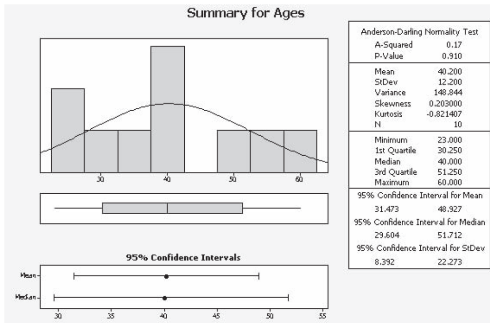
FIGURA 2-21 Pantalla de Minitab de Graphical Summary
