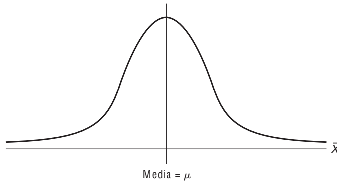
FIGURA 2-8 Distribución muestral de \bar{X}
