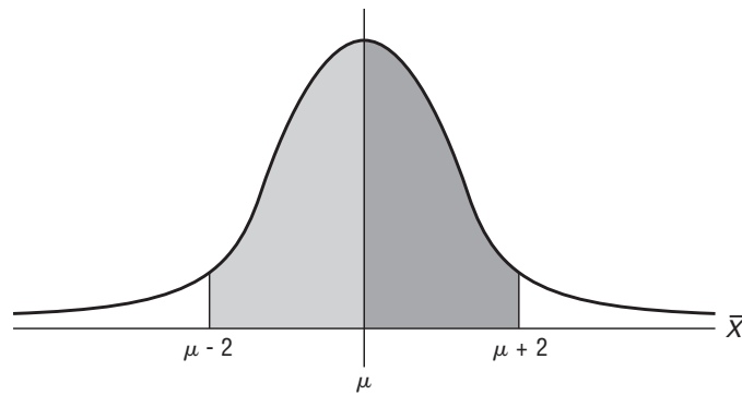
FIGURA 2-9 Áreas de distribución muestral para el ejemplo 2.5
